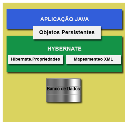
Figura 20 – Mapeamento Hibernate
